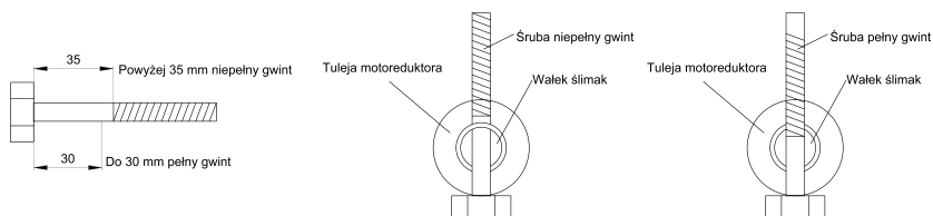
Rysunek 2. Rysunek śruby zalecanej przez producenta
